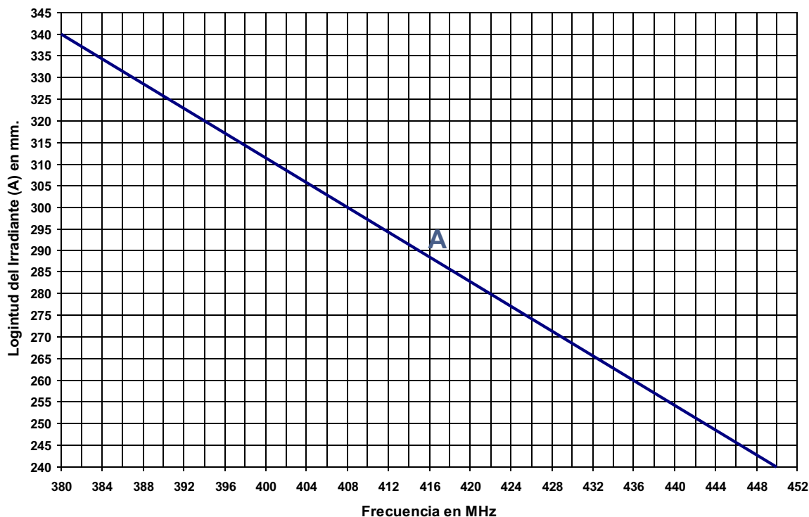
Corte Aproximado
